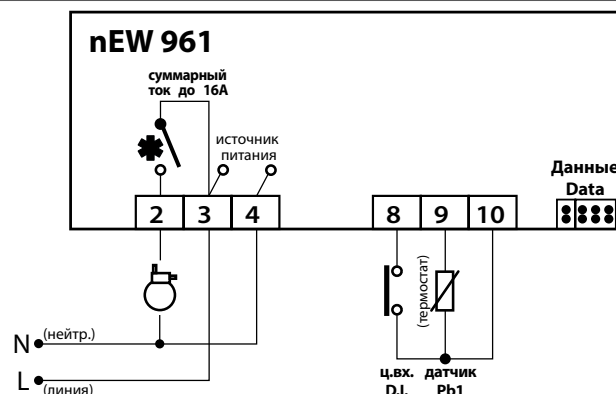
nEW 961 с блоками винтовых клемм
