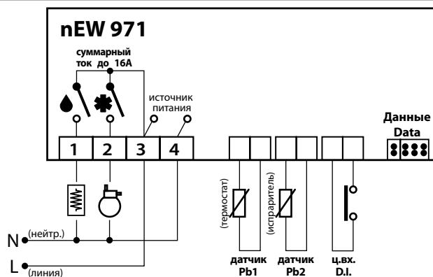
nEW 971 с быстрозъемными разъемами типа FastOn
