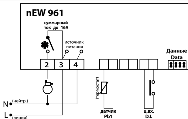
nEW 961 с быстрозъемными разъемами типа FastOn
