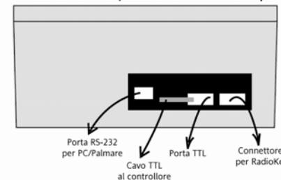
Box Elettrico con interfaccia RS-232/TTL RadioAdapter
