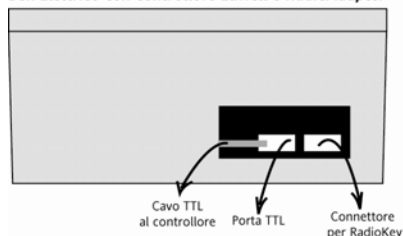
Box Elettrico con controllore Eliwell e RadioAdapter
