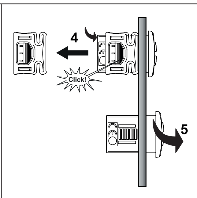
Рис. 10. Пример снятия
