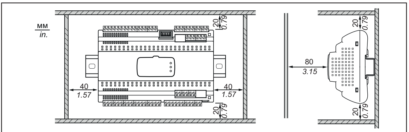
Рис. 6. Расстояния
