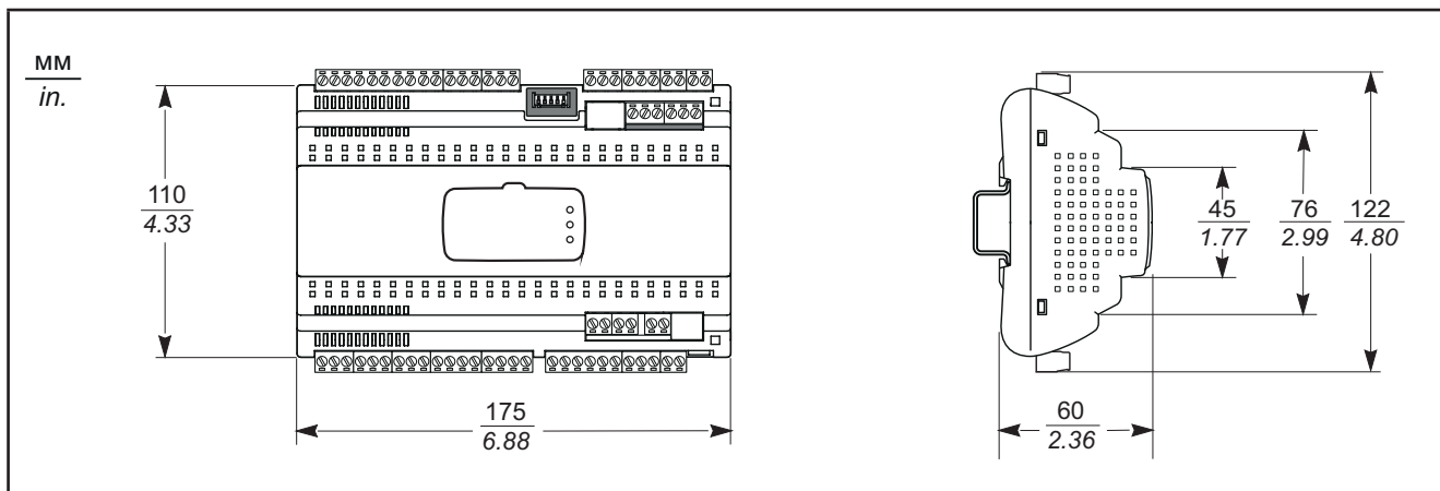
Рис. 36. Механические размеры
