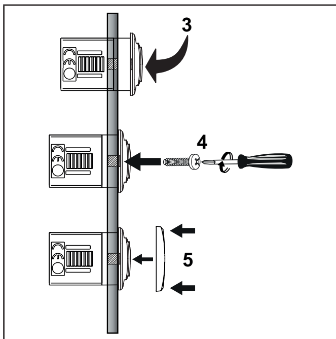
Рис. 13. Пример установки
