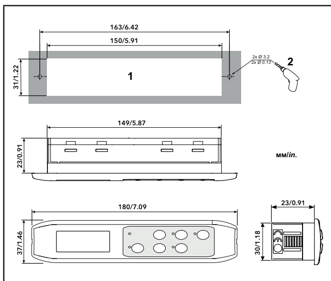
Рис. 11. Размеры
