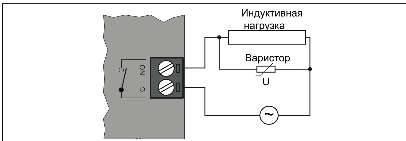
Рис. 29. Защитная цепь типа В
