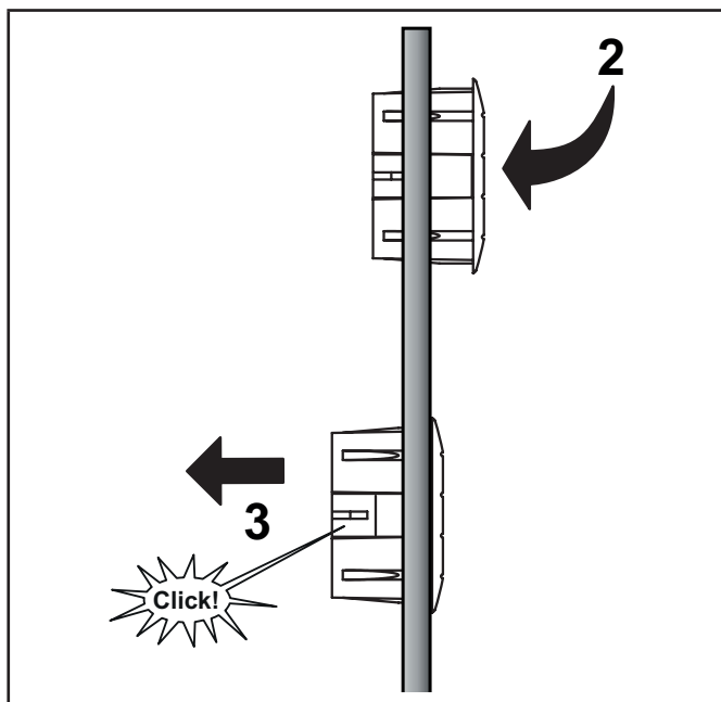
Рис. 23. Пример установки
