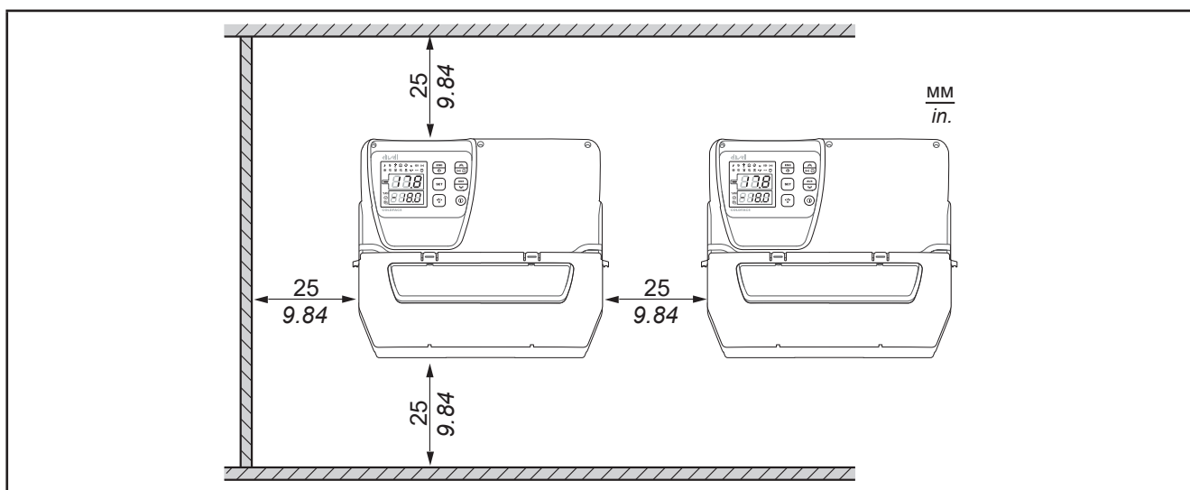
Рис. 1. Требования по расстояниям, применимые ко всем моделям
