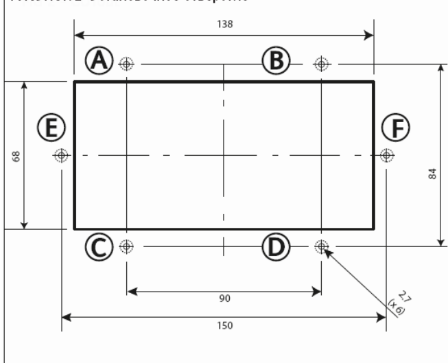
РИСУНОК 2 Установочное отверстие
