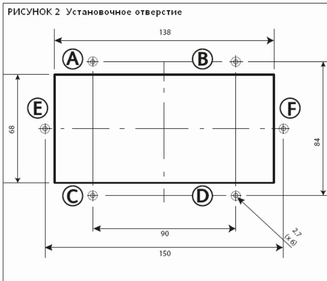
РИСУНОК 2 Установочное отверстие
