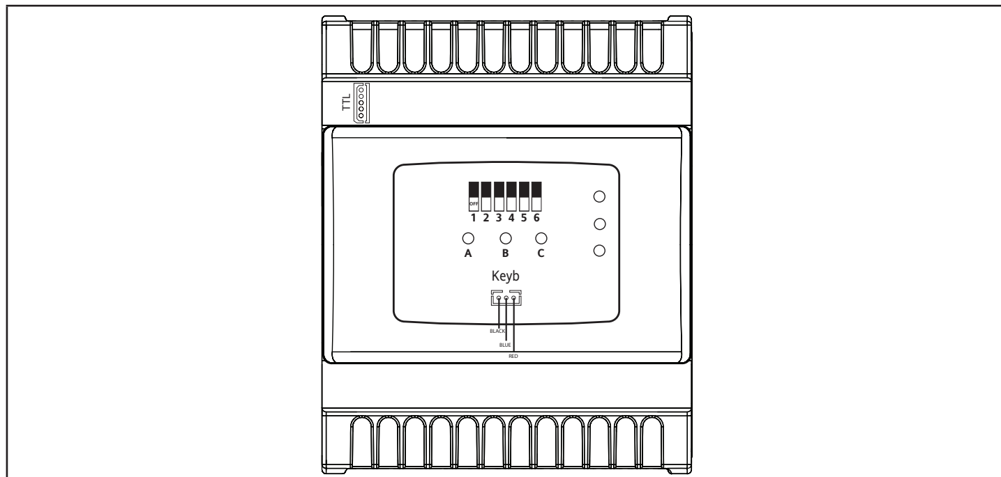
Рис. 20 Подключение Мультифункционального ключа (МФК)
