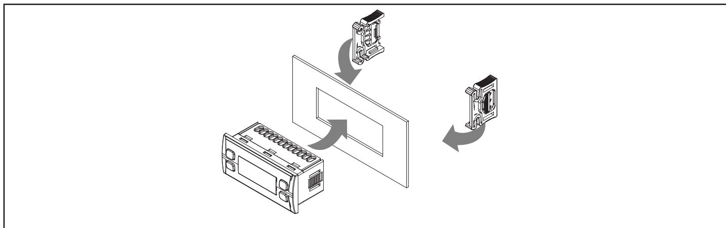
Рис. 5 Установка SKP 10
