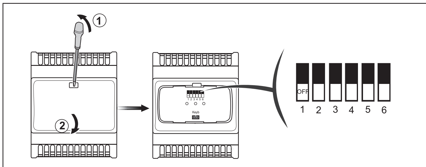
Рис. 4 Доступ к DIP переключателям/разъему SKP 10 - 1
