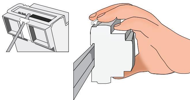
Рис. 3 Пример установки на DIN рейку - Вид 3/4
