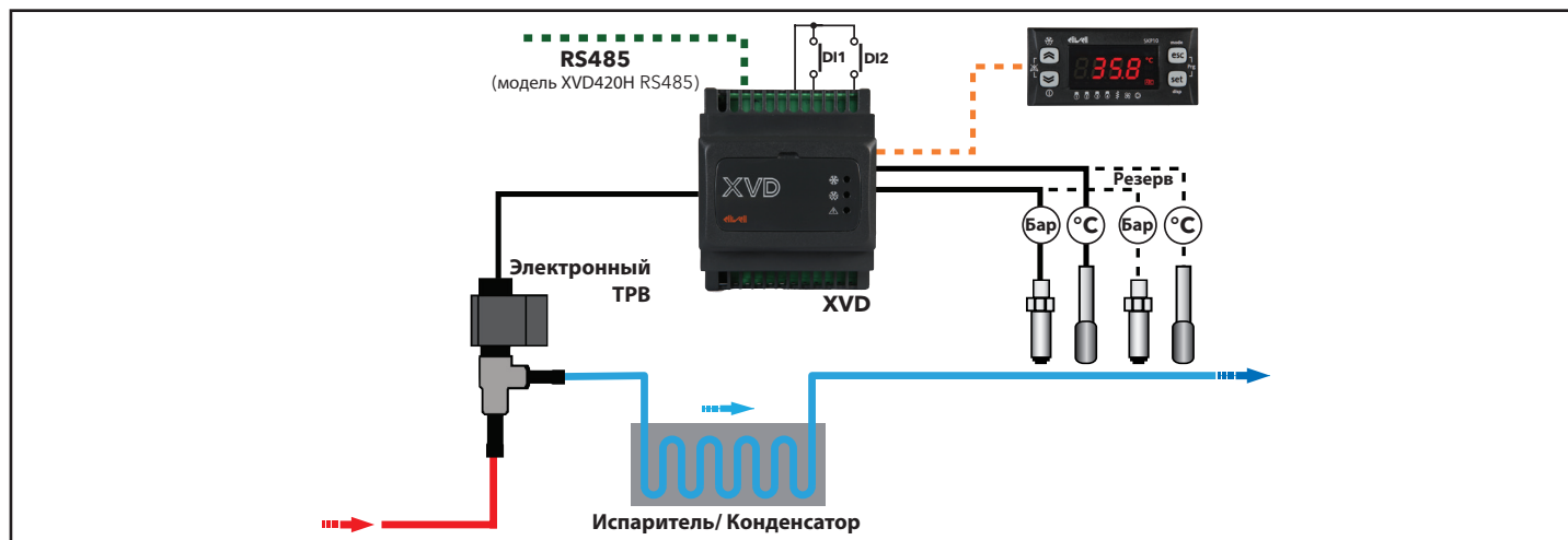
Рис. 19 Применение - Отдельно стоящий драйвер
