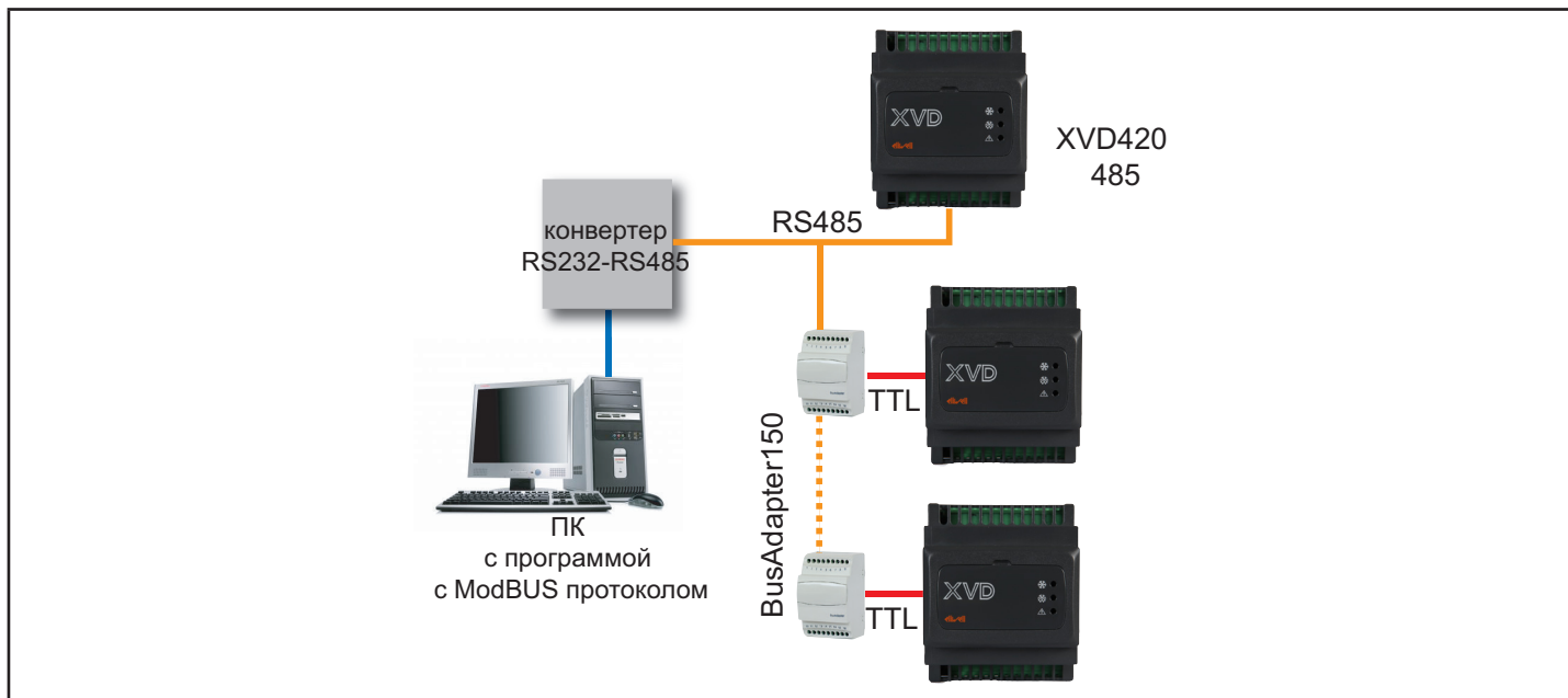
Рис. 22 Подключение по ModBus к группе приборов по шине RS485
