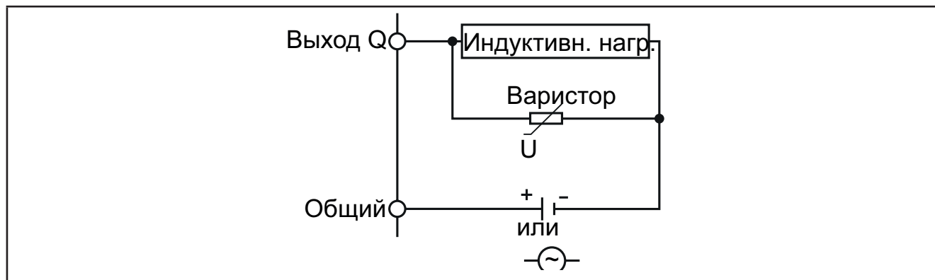
Рис. 8 Защитная цепь С
